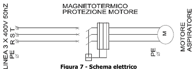
Figura 7 - Schema elettrico
