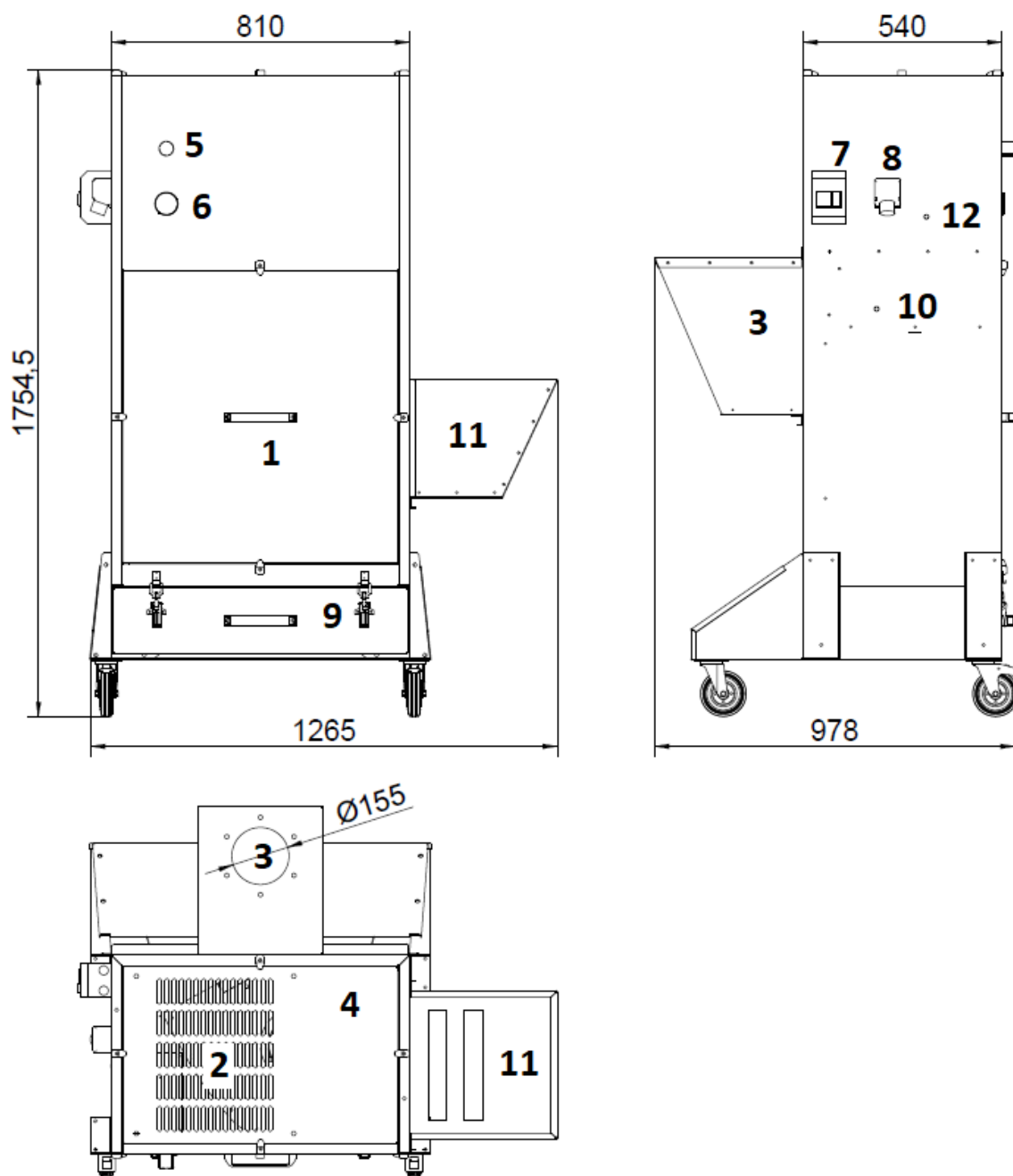
Figura 2 - Quote di riferimento DFC11NBTX
