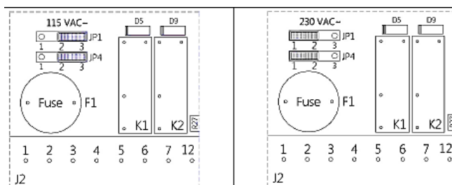
Figura 11 - Configurazione dei ponticelli ingresso 115V o 220V
