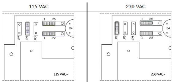
Figura 12 - Configurazione ponticelli uscita 115 Vac e 220Vac
