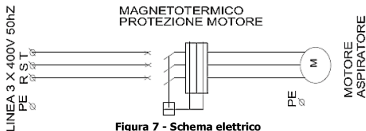
Figura 7 - Schema elettrico
