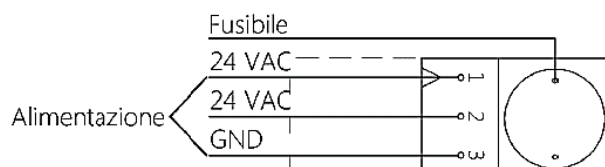
Figura 9 - Collegamento centralina 24Vac
