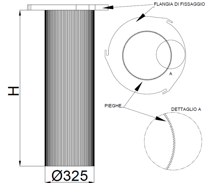
Figura 3 - Cartuccia
