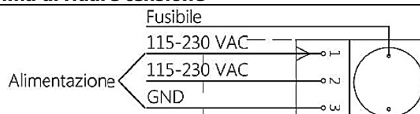
Figura 8 - Collegamento Centralina 115/230V
