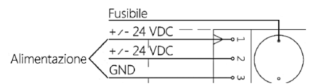
Figura 10 - Collegamento centralina 24Vdc
