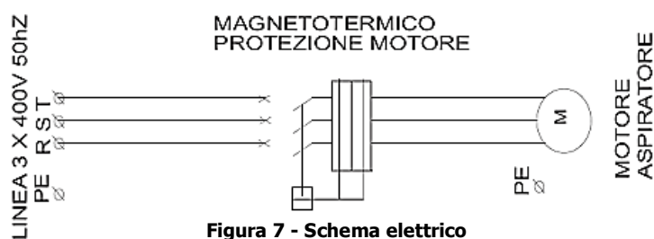
Figura 7 - Schema elettrico
